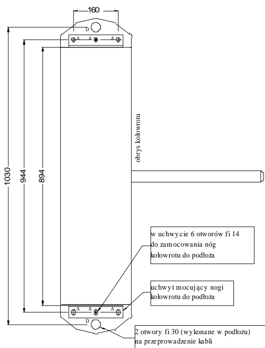
LK715 - owiert podłoża
