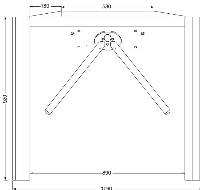
LK715 - widok z boku
