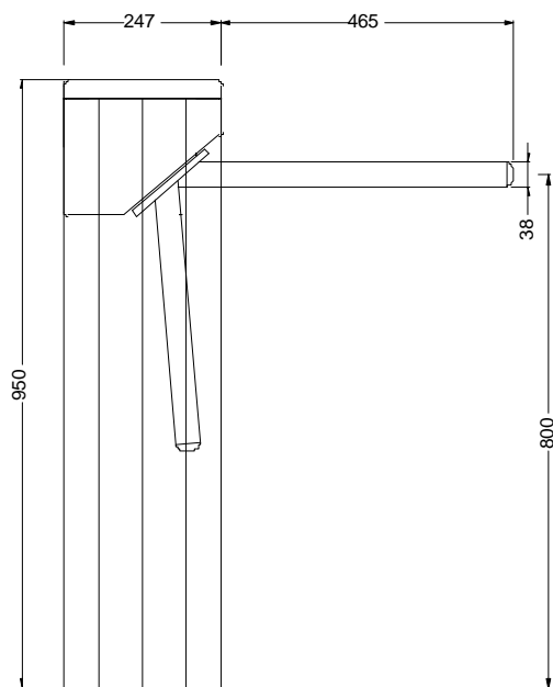
LK715 - widok od strony przejścia
