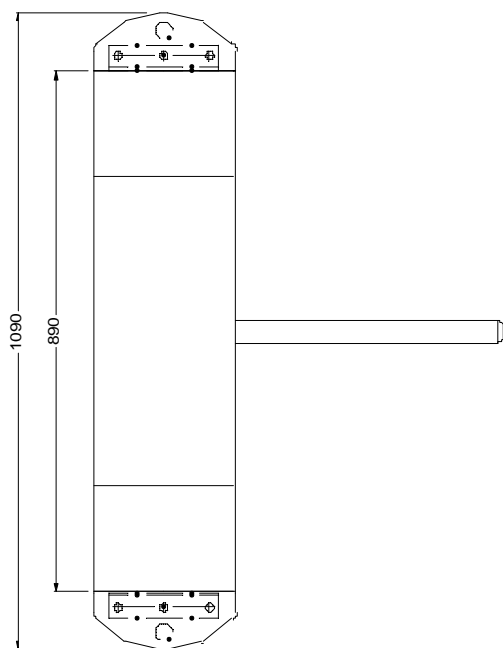
LK715 - rzut pionowy
