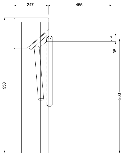
LK516 - widok od strony przejścia
